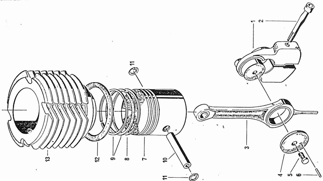
Bildtafel 2: Triebwerk - Kolben - Zylinder table 2: gearing - piston - cylinder tableau 2: embiellage - piston - cylindre
